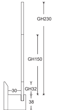
H 70 D 54 L 250/500/1000/1500/2000 GH = glashöjd / glass height
