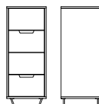
H 1169 B 460 D 450
