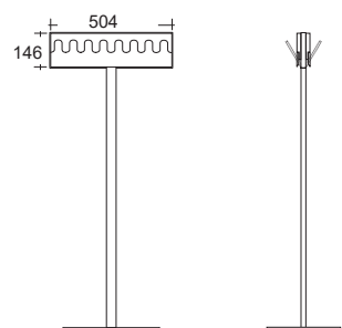
H 1250/1650 B 400 D 305
